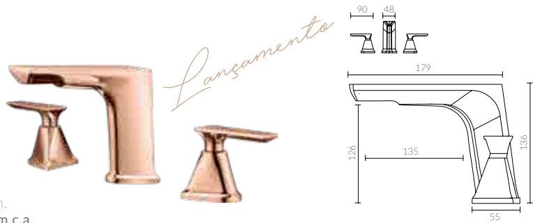
Ref. RB8894 Misturador duplocomando para lavatório. Acabamento rose gold.
